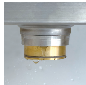
地漏芯關閉防臭
