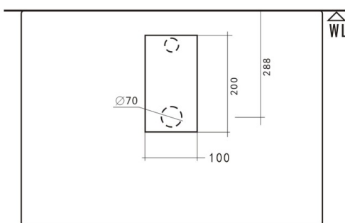
面盆開孔圖
